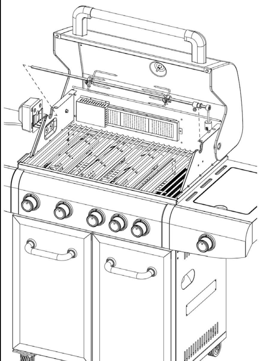
Insert Rotisserie Rod
